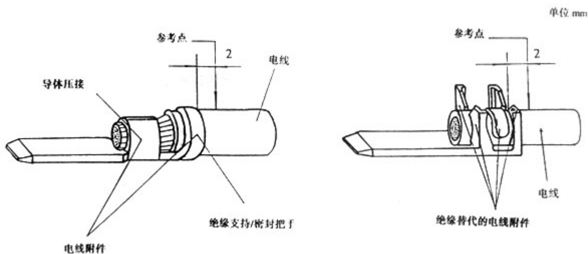
图 1 插头
