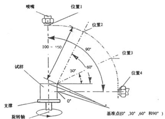
图 11 试样放置
