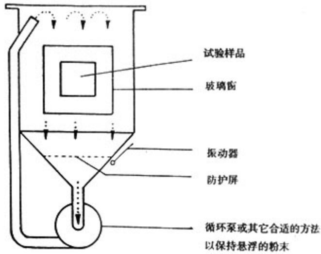
图 18 灰尘试验
