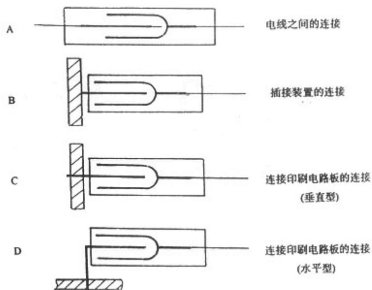
图 3 连接举例
