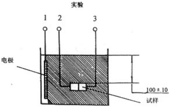
图 8 水密性试验
