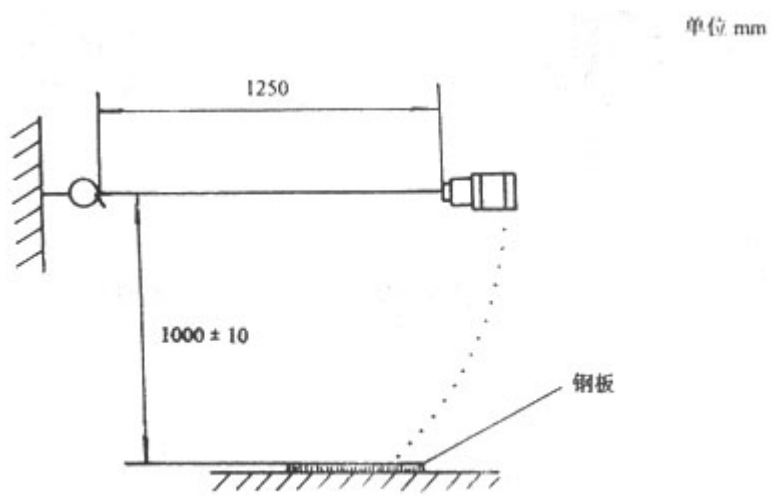
图 17 下落试验安排
