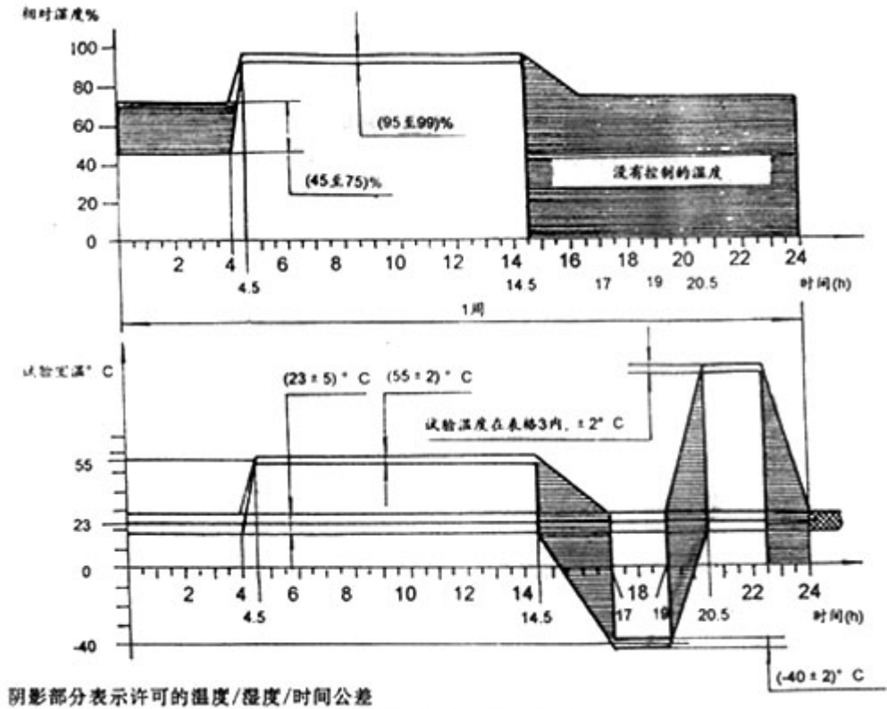
图 12 温度/湿度循环
