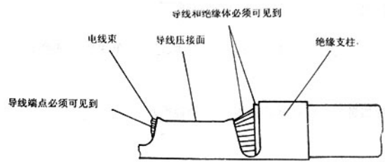
图 5 导线与插接件的压接连接
