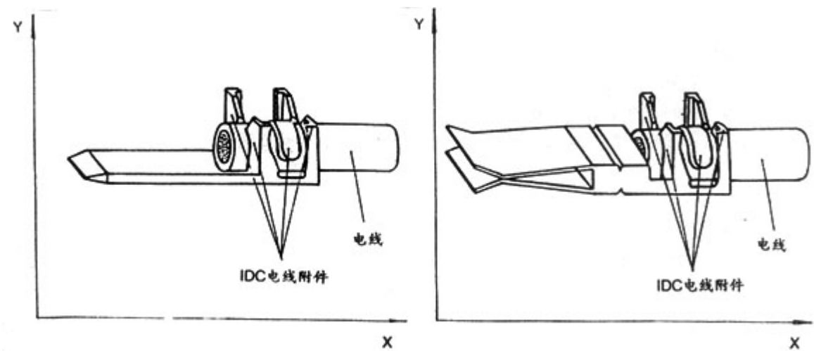
图 B1 IDC 电线附件抗拉力测试
