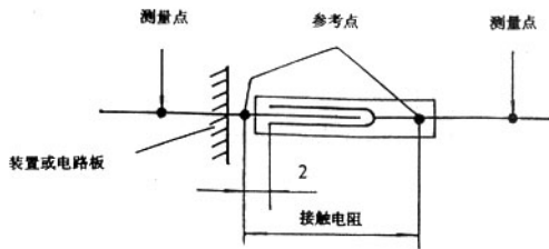
图 7 接触电阻(电器连接)
