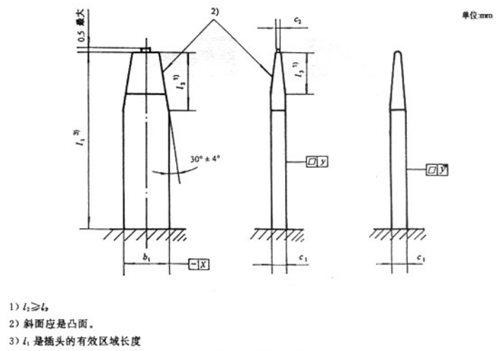
图 1 插头尺寸
