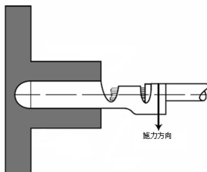
图 2 端子弯曲强度测试
