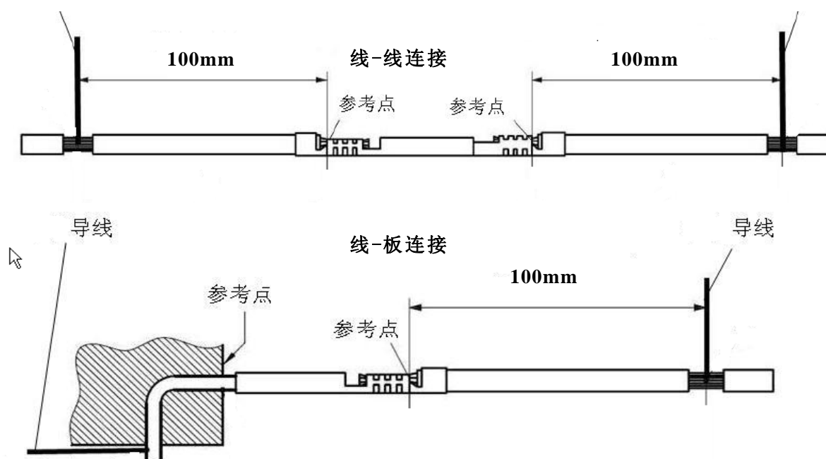
图 7 接触电阻测试
