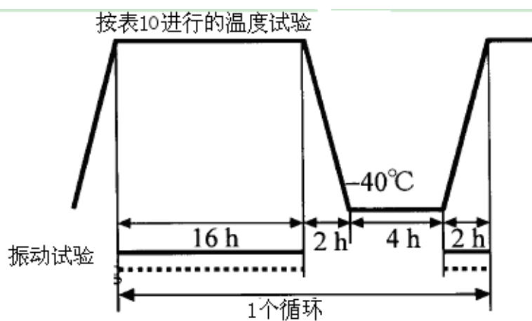
图 14 复合环境测试循环
