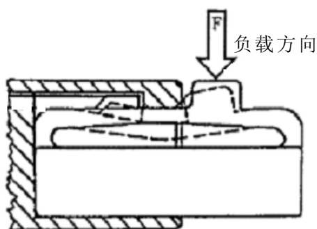
图 4 解锁力测试
