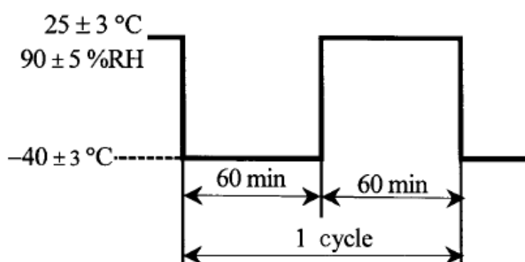
图 17 结露试验循环
