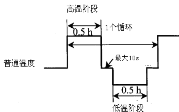
图 13 循环周期
