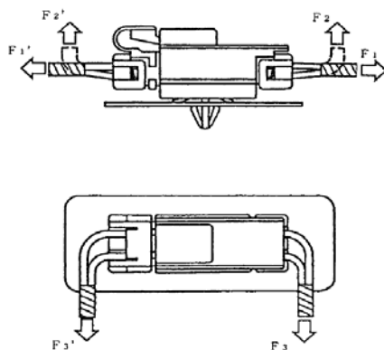
图 5 连接器卡扣离脱力测试
