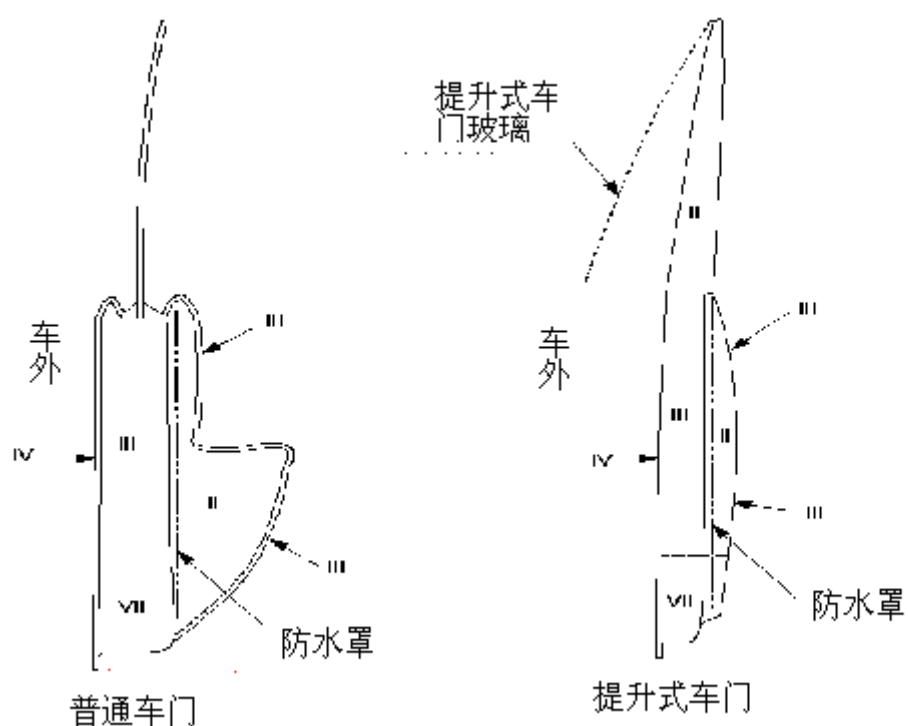
图 C.2 车门不同部位的防水等级
