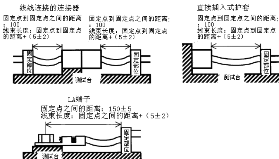
图 10 振动测试样品安装
