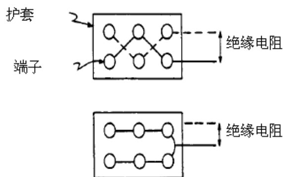
图 9 绝缘电阻测试
