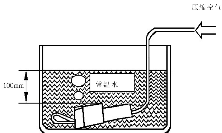
图 6 密封性测试
