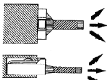
图 3 锁合力测试
