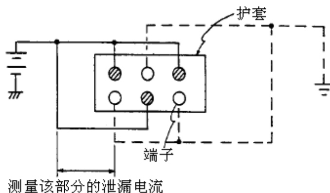
图 16 防潮测量装置
