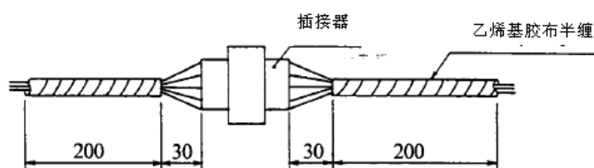
图 8 温升测试
