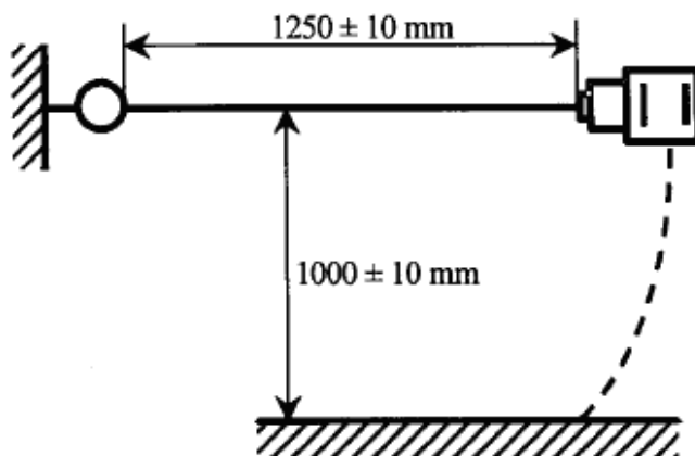
图 12 跌落冲击测试
