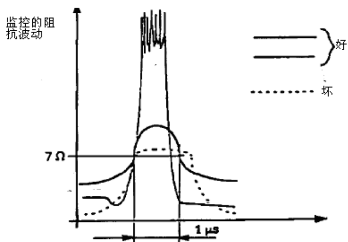
图 11 振动试验中的阻抗
