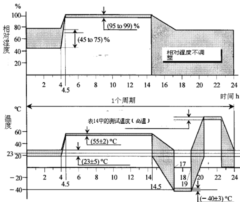
图 15 温湿度循环测试
